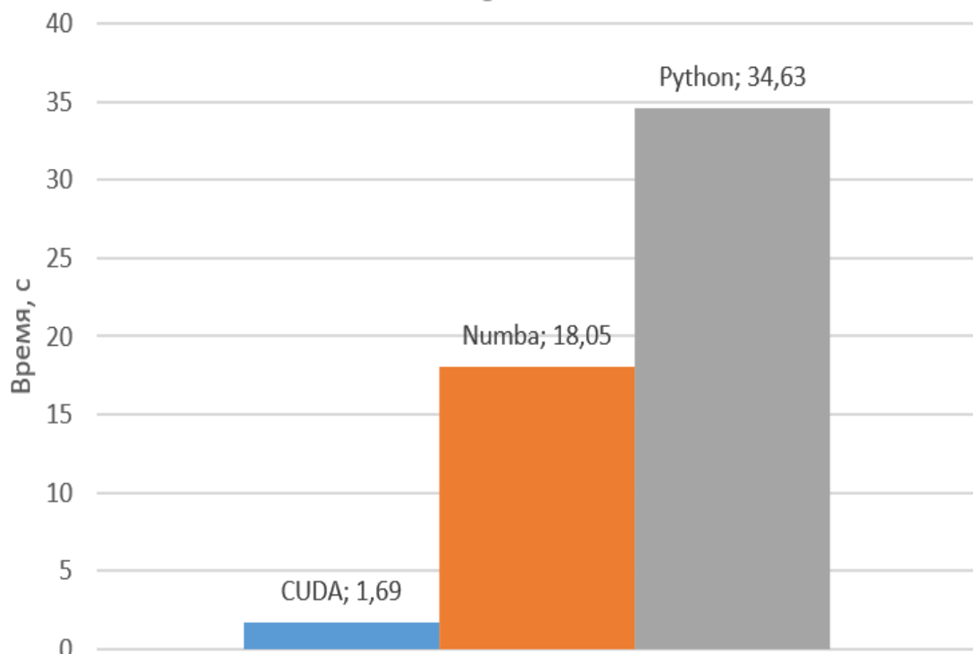
Время построения изображения 50 × 50 пикселей
