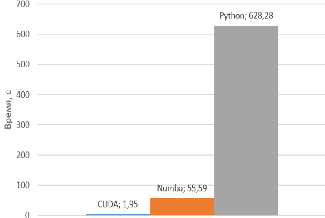
Время построения изображения 150 × 150 пикселей
