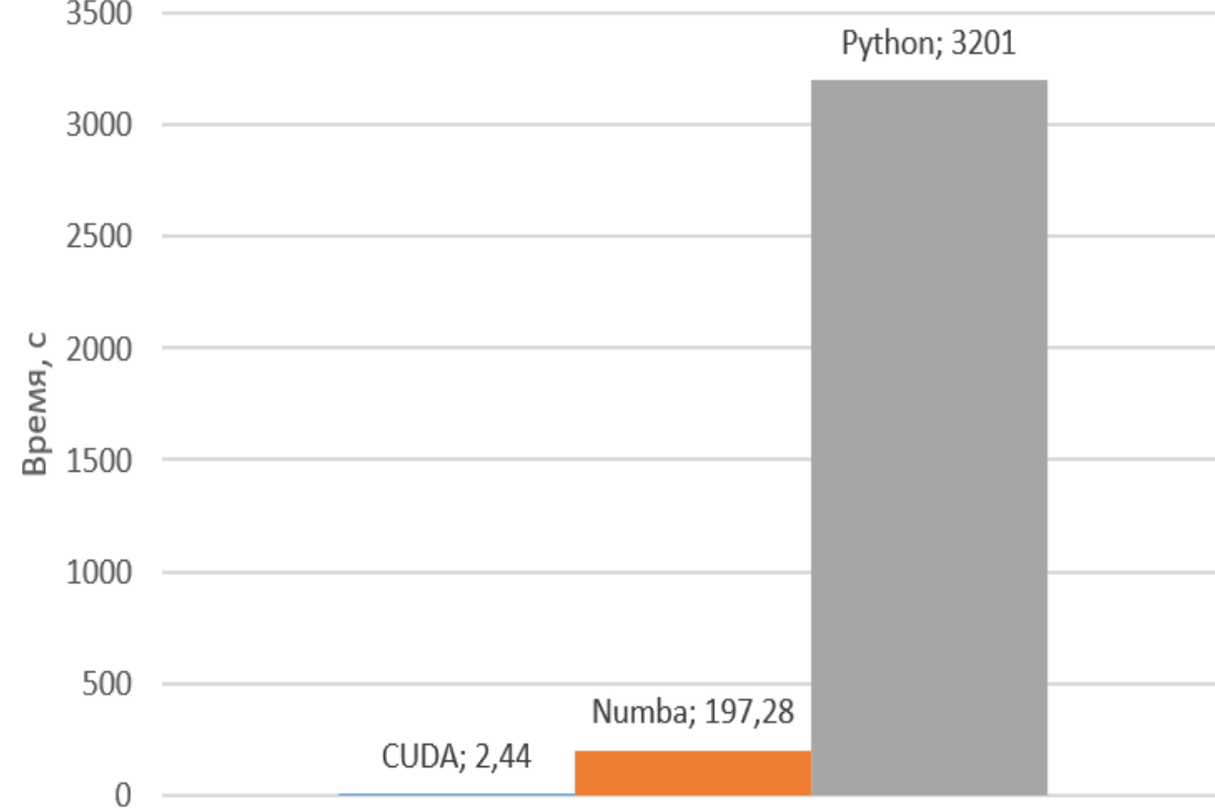
Время построения изображения 300 × 300 пикселей
