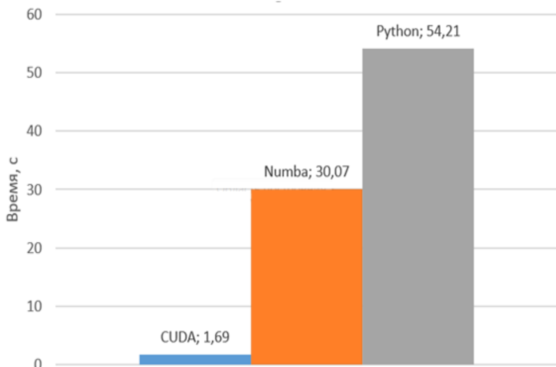
Время построения изображения 100 × 100 пикселей
