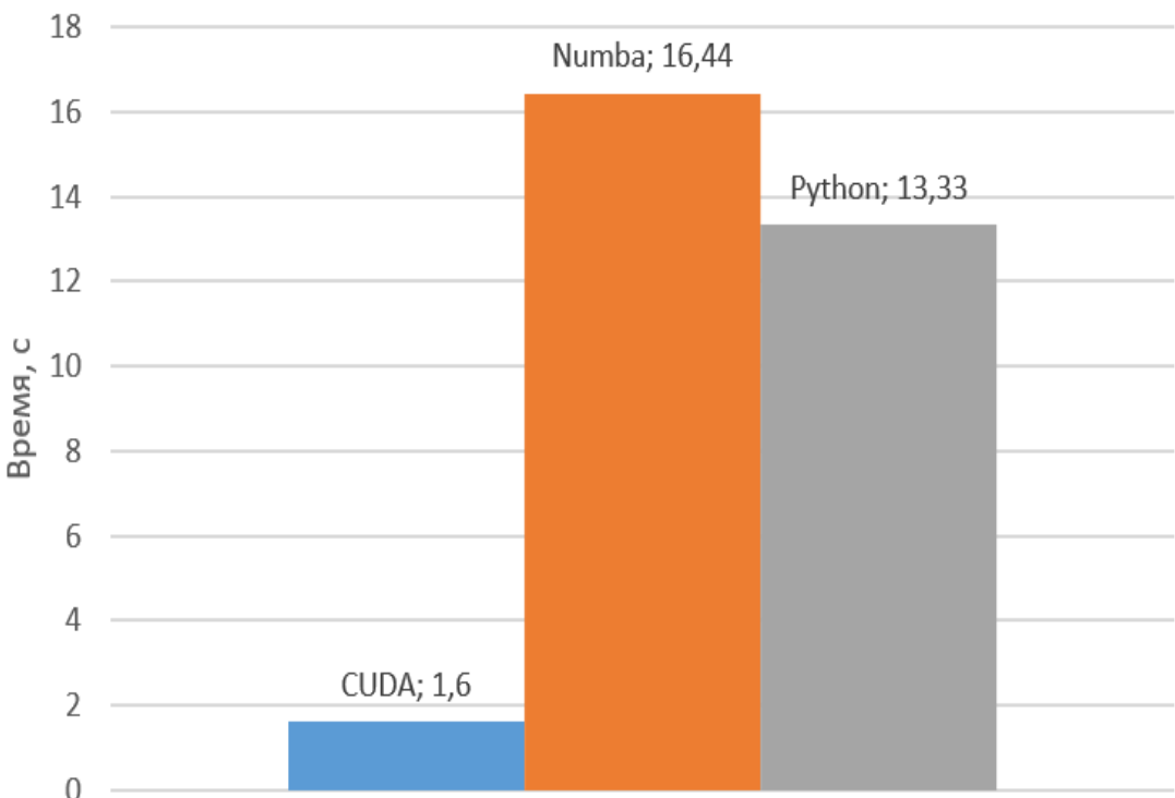
Время построения изображения 20 × 20 пикселей
